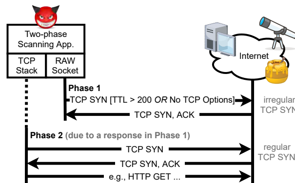
Abbildung 5.11: Zwei-Phasen Scanner.
