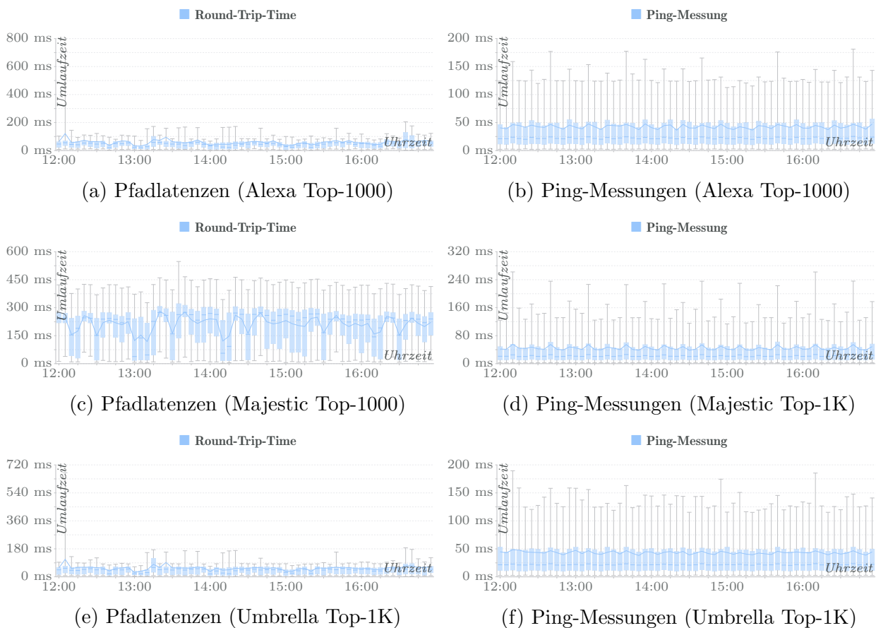
Abbildung 2.62: [I13] Pfadanalyse , Messziele in DNS-Toplisten (Data Plane)
